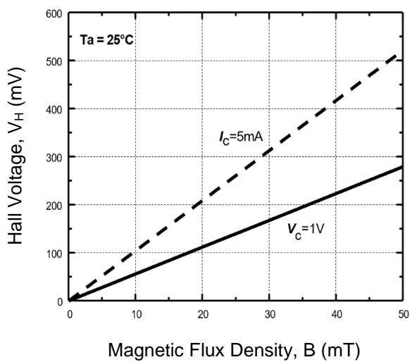
Fig.2 V_H - B
